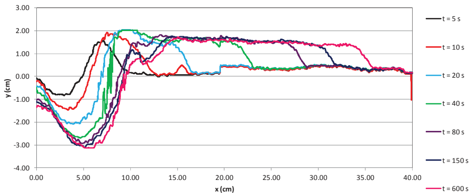
Fig. 5. Time evolution of the sediment bed in case of test condition N.1.
