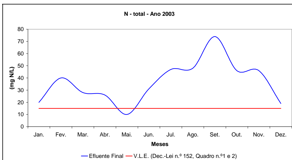
Figura 10 – Evolução do azoto no ano 2003, desde a entrada na ETAR até à saída.
