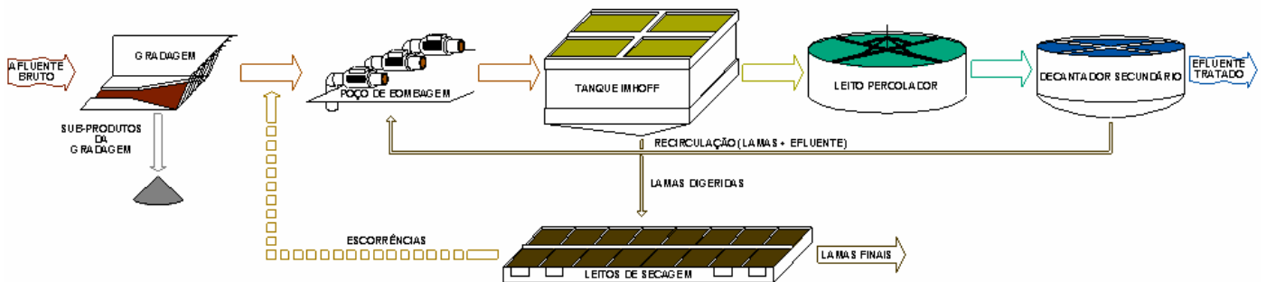
Figura 6 – Fluxograma da ETAR de Ponte de Lima.
