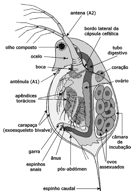
FIGURA 1. Representação esquemática da anatomia interna e externa de uma pulga-de-água ( Daphnia sp.).
