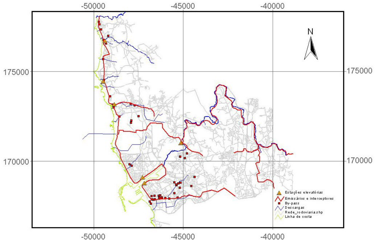
Figura 4 – Emissários e interceptores, estações elevatórias e by-pass do concelho de Matosinhos.
