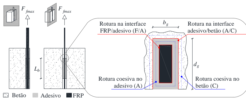
Figura 1. Exemplo de ensaio de arranque direto e possíveis modos de rotura locais.
